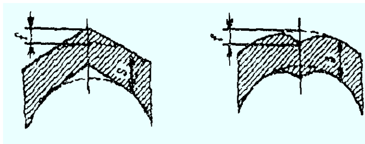
Рис. 1. Увод (угловатость) кромок в сварных швах
